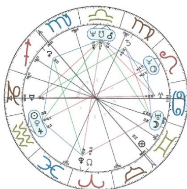
Karen Rosenkilde ma 30. jan 1950 kl. 07:20:00 i København, Danmark +01:00 CET (Europe/Copenhagen) 55°40'33" N 12°33'56" E
