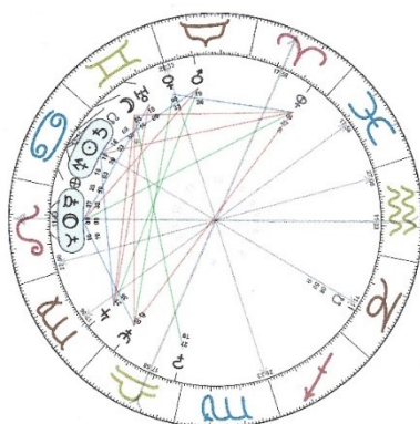
Niels Arthim Skriver sø 8. jul 1945 kl. 07:12:53 i København, Danmark +02:00 CEST (Europe/Copenhagen) 55°40'33" N 12°33'56" E
