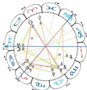
Composithoroskop for Niels & Karen
